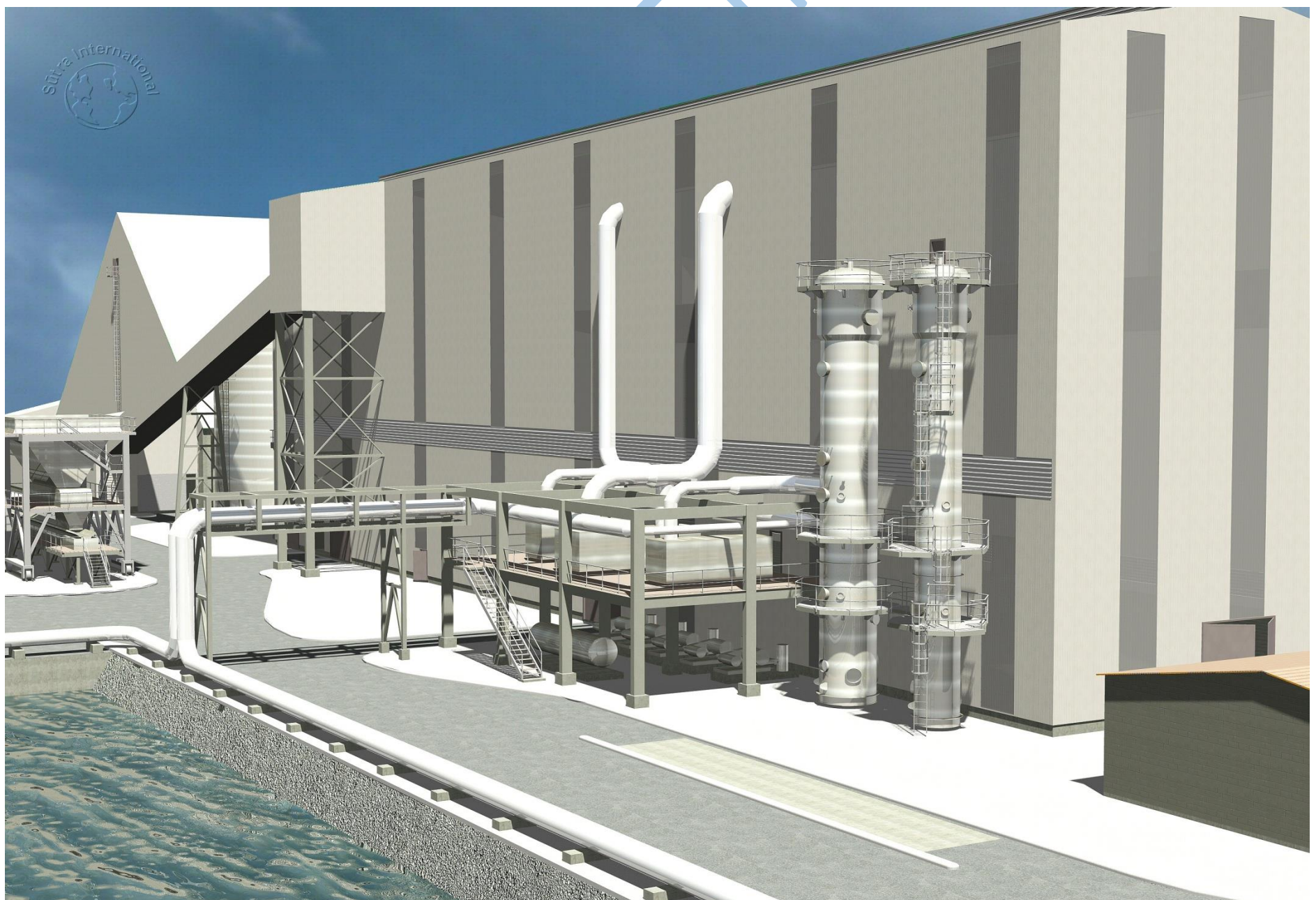
✚ Vue d'arrière concentrateur-utilité (Tunisie Sucre) :
